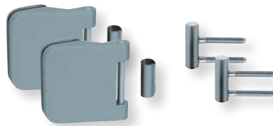
Glastürset Form A Blind mit 3-teiligen Glastürbändern abgerundet, abgesetzter Falle und Rahmenteilen für Holzzargen. EDELSTAHL matt
