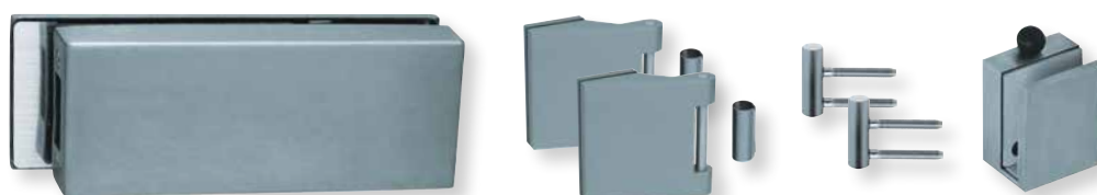
Standflügelset Form B Gegenkasten lang mit 3-teiligen Glastürbändern eckig, Rahmenteil für Holzzargen und Türfeststeller. EDELSTAHL matt
